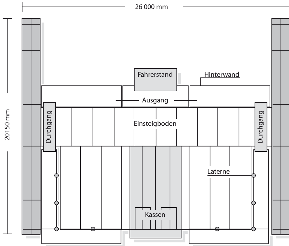
Grundriss
